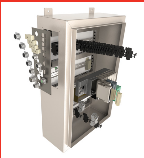
Armoire électrique de GLSV, rendu éclaté de SOLIDWORKS Electrical
